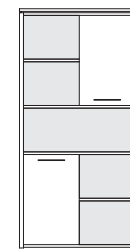
Elemento c/ prateleiras 2 portas madeira Module with shelf 2 wood doors A 185,5 x L 90 x P 40
